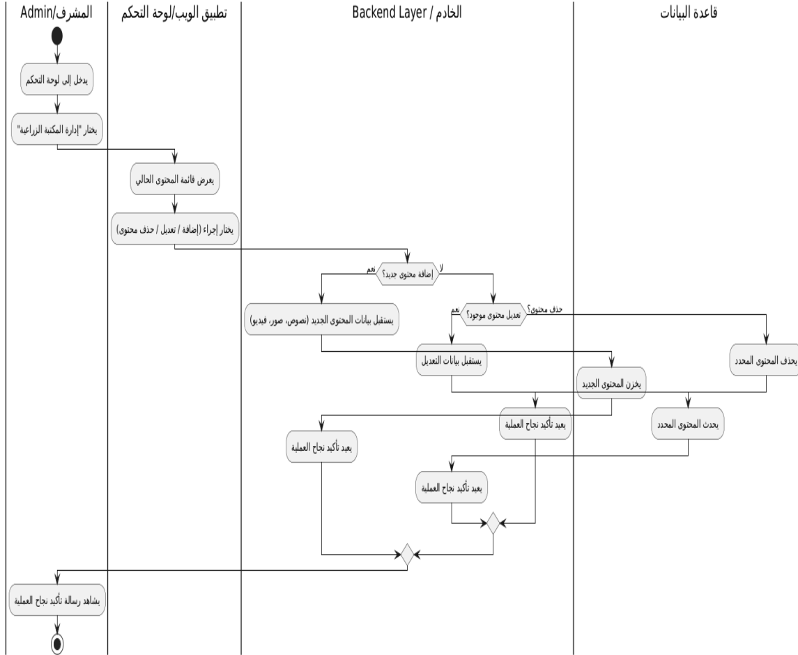
رسم توضيحي 9-1: مخطط النشاط إدارة المكتبة الزراعية
