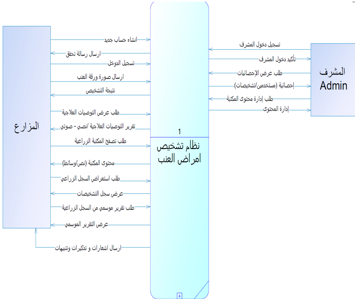
رسم توضيحي 1-2 : مخطط السياق (Context)
