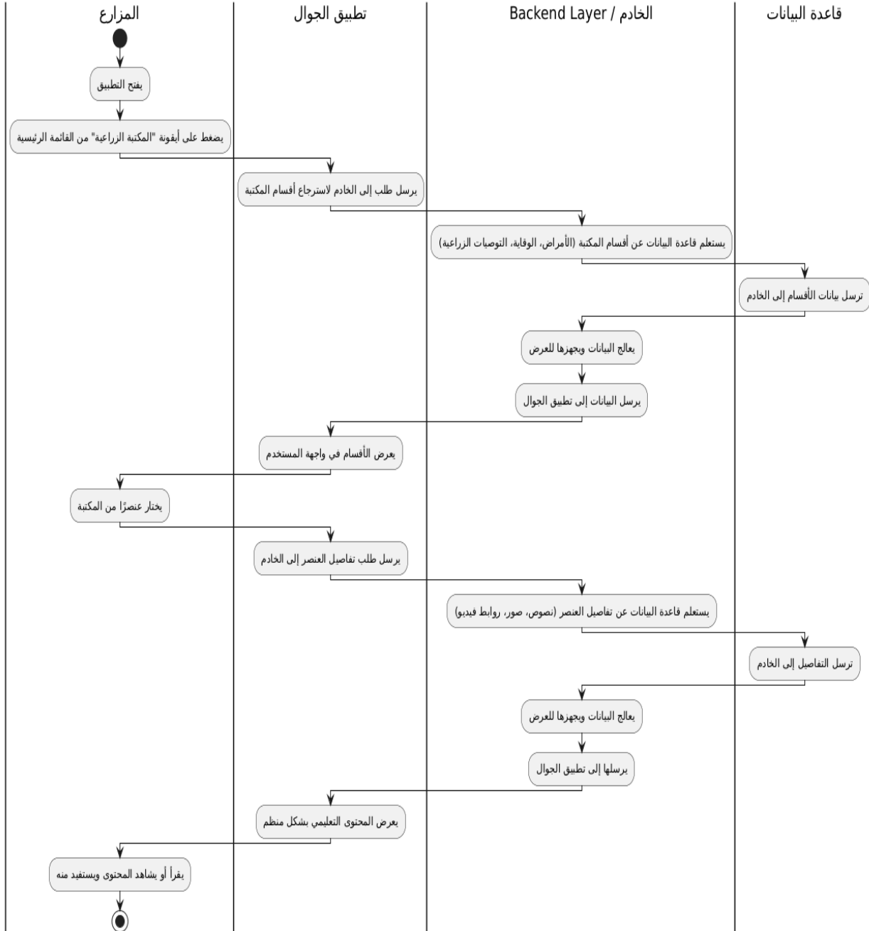
رسم توضيحي 7-1: مخطط النشاط تصفح المكتبة الزراعية
