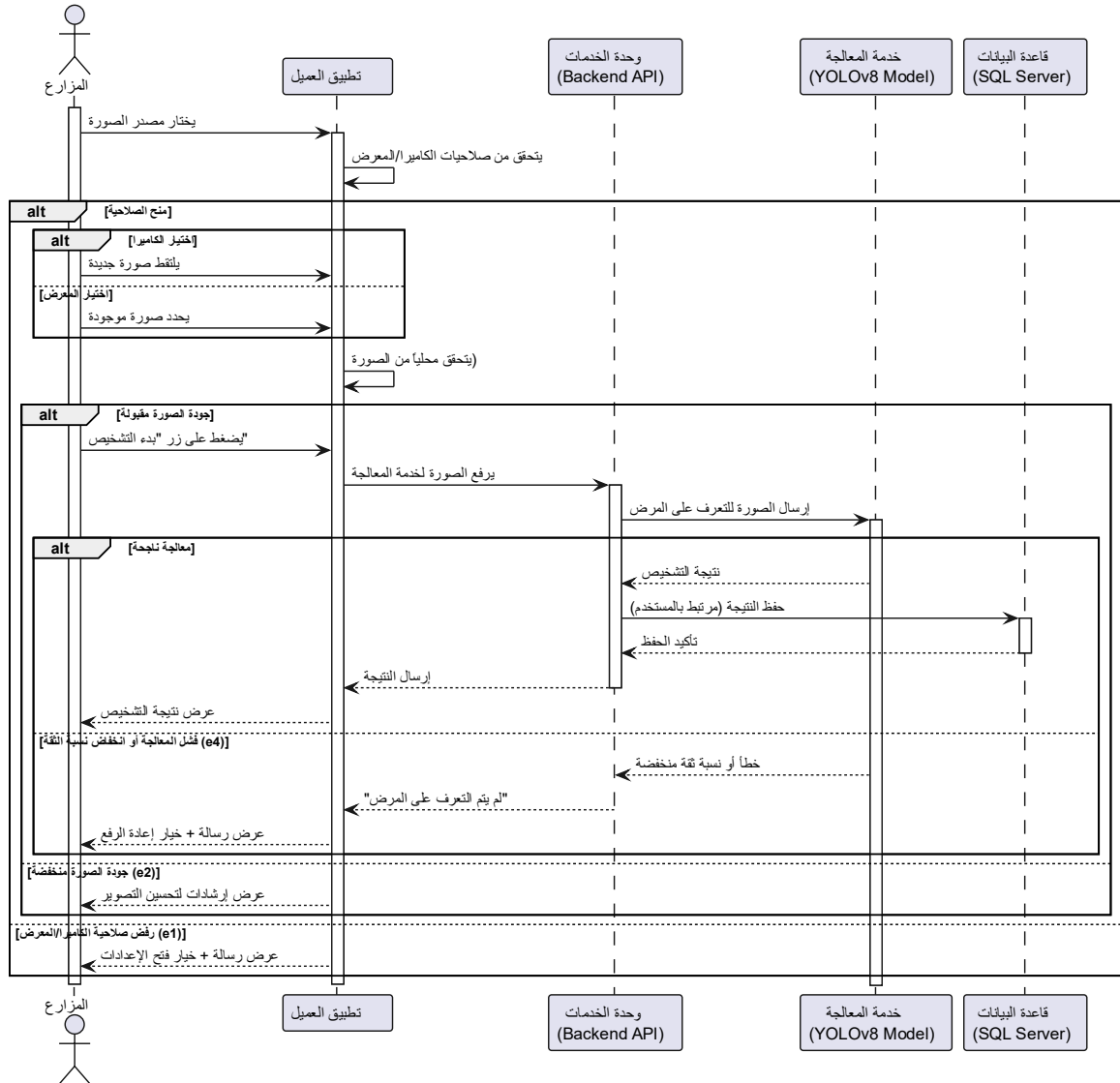
رسم توضيحي 1-10: مخطط رفع الصورة والتشخيص
