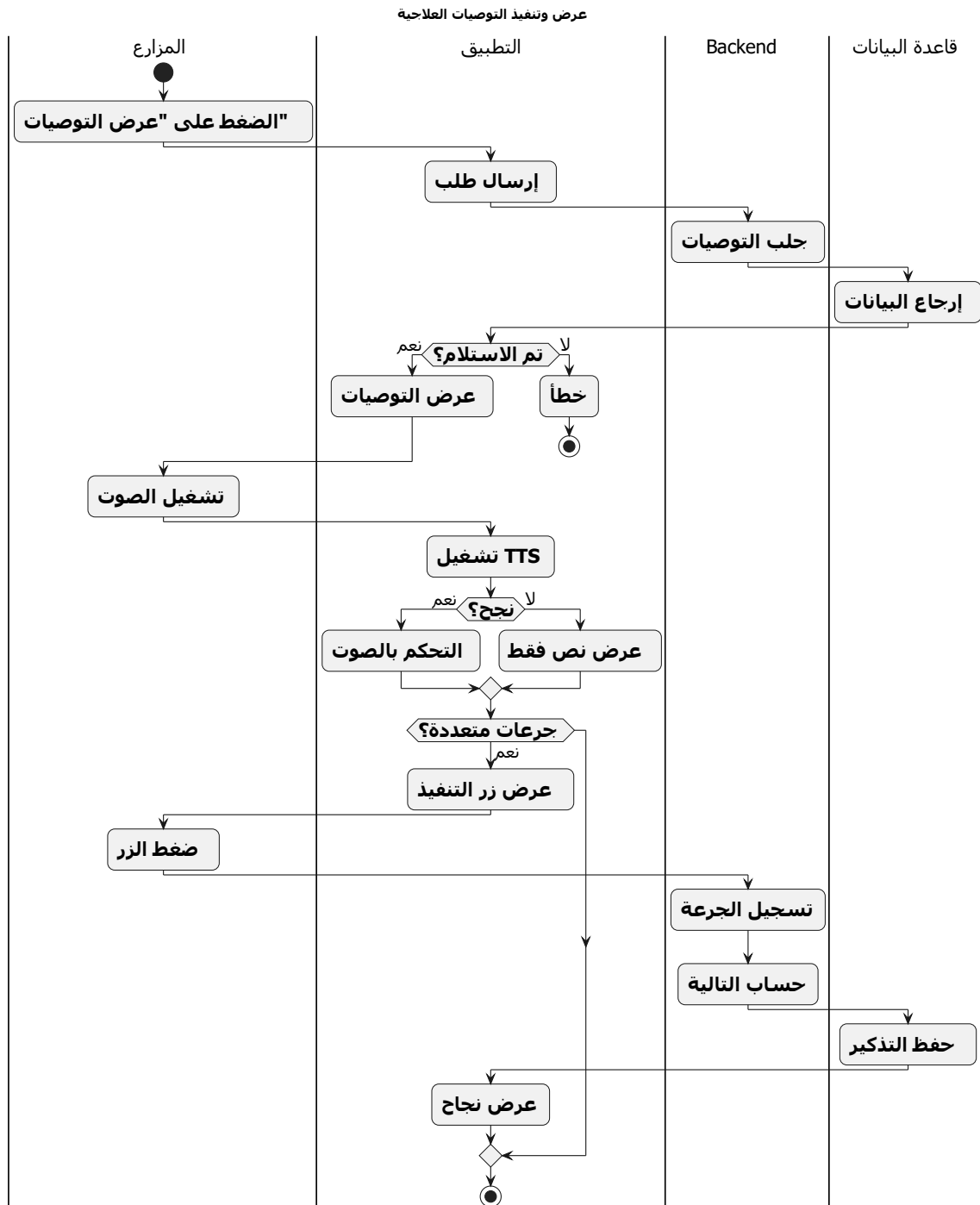
رسم توضيحي 1-5: مخطط النشاط عرض وتنفيذ التوصيات العلاجية
