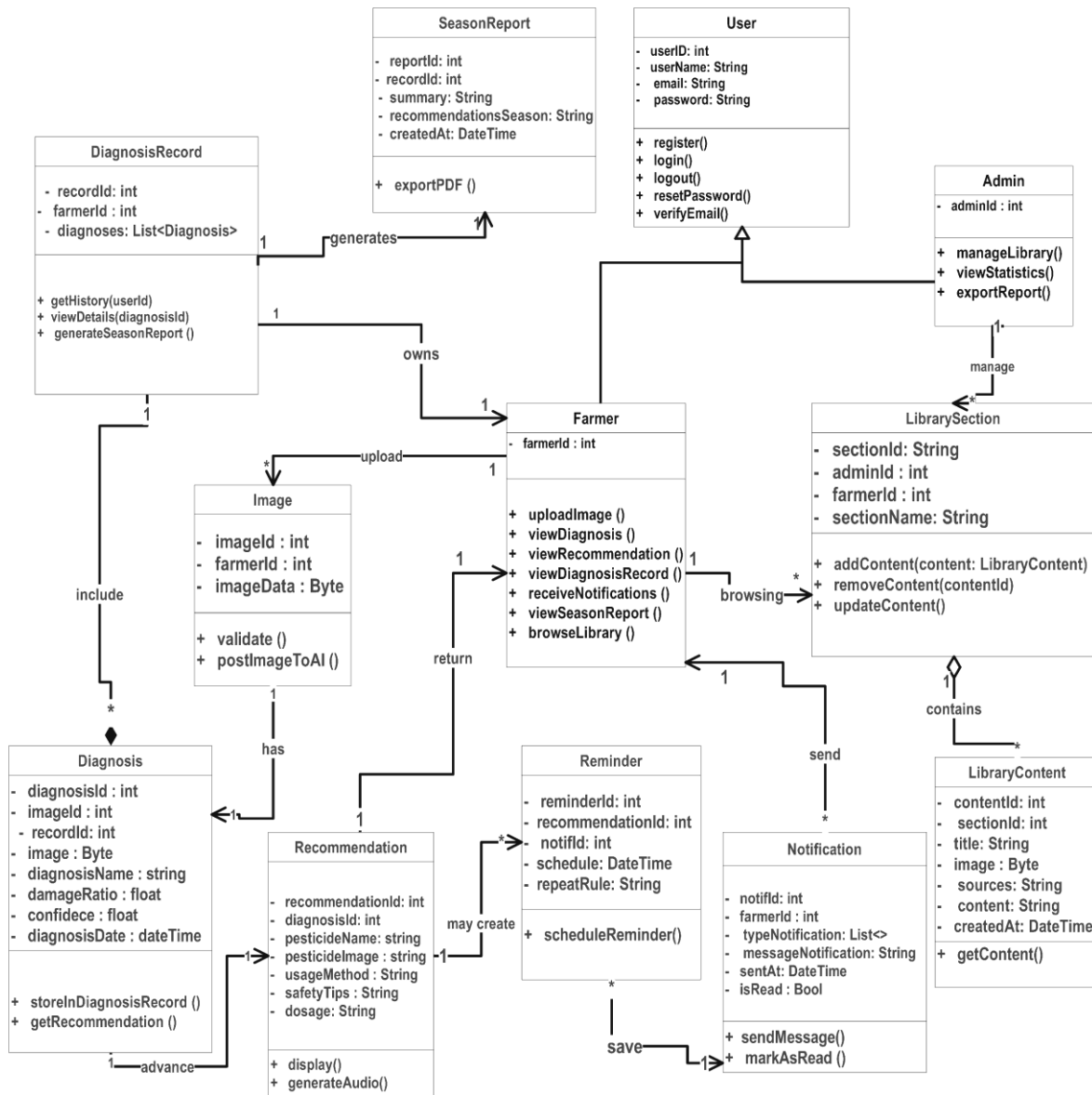
رسم توضيحي 1-16: مخطط الكلاس (Diagram Class)
