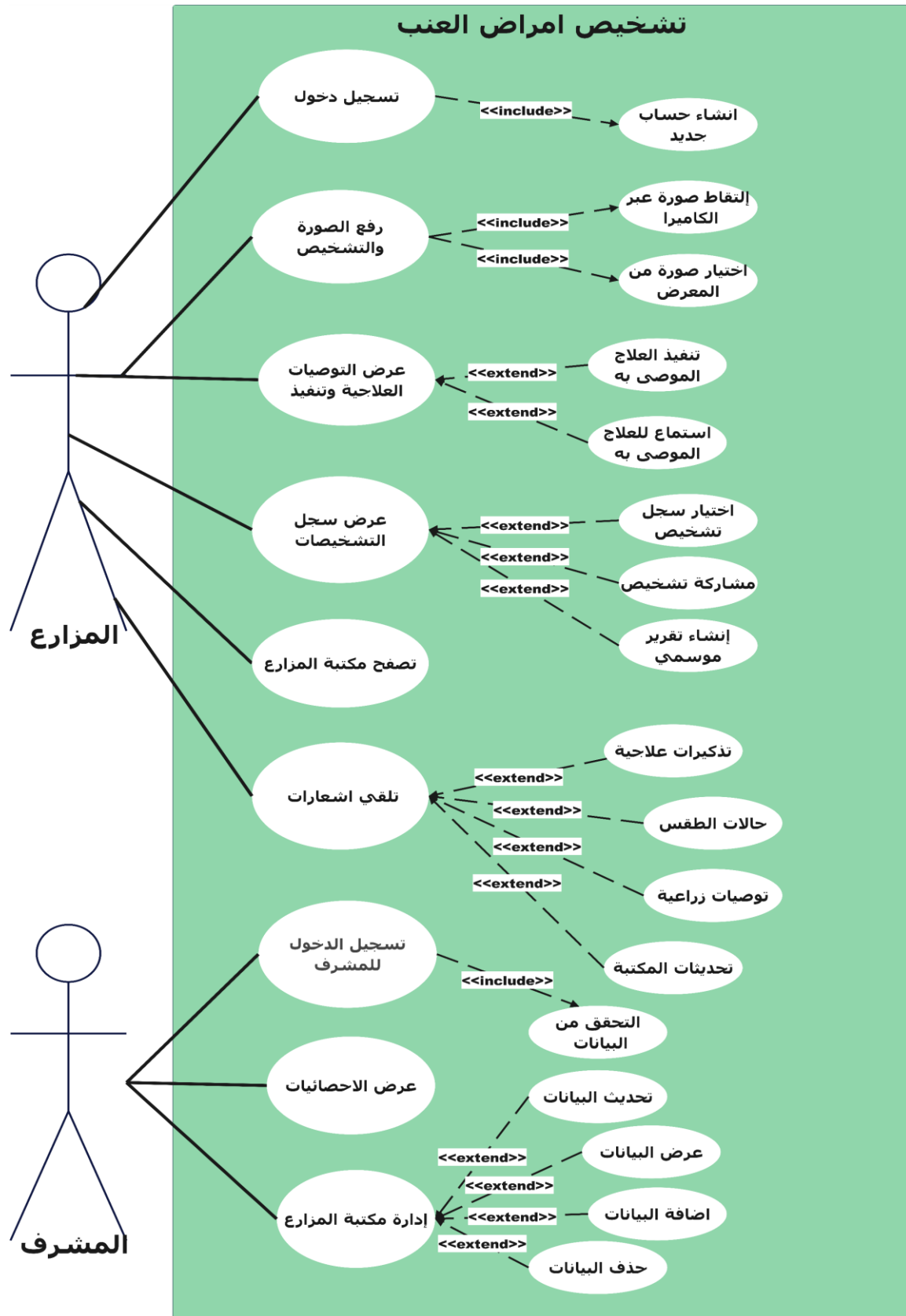
رسم توضيحي 1-3: مخطط حالة الاستخدام (Use Case Diagram)
