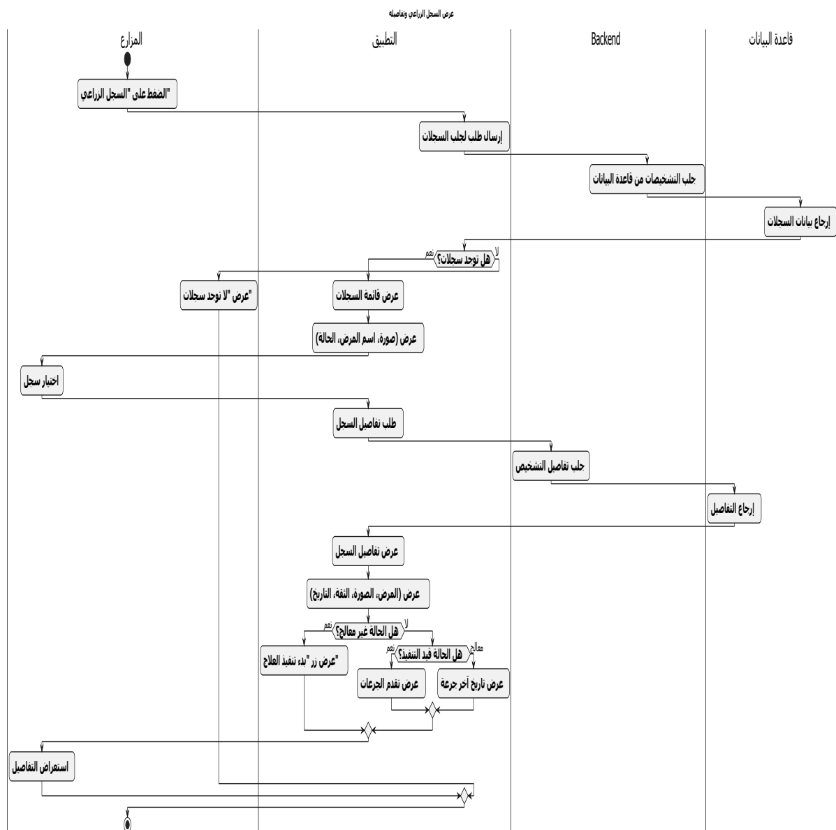
رسم توضيحي 1-6: مخطط النشاط عرض السجل الزراعي وتفصيله
