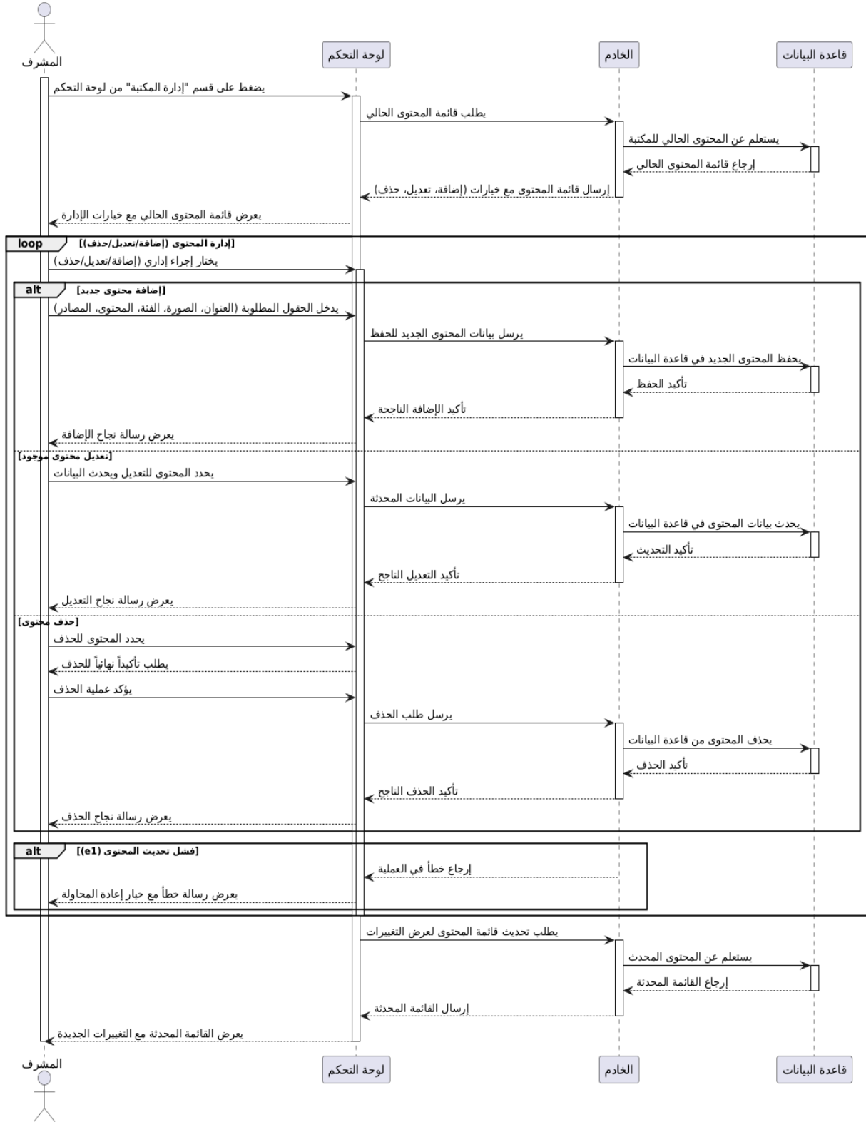
رسم توضيحي 1-15: مخطط إدارة المكتبة الزراعية
