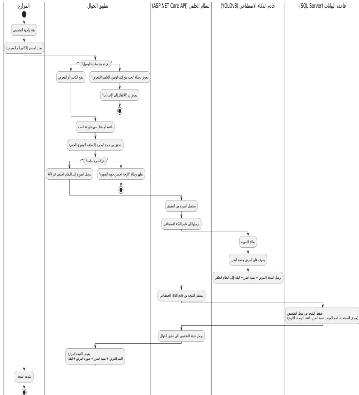
رسم توضيحي 1-4: مخطط النشاط لعملية رفع الصورة وتشخيص
