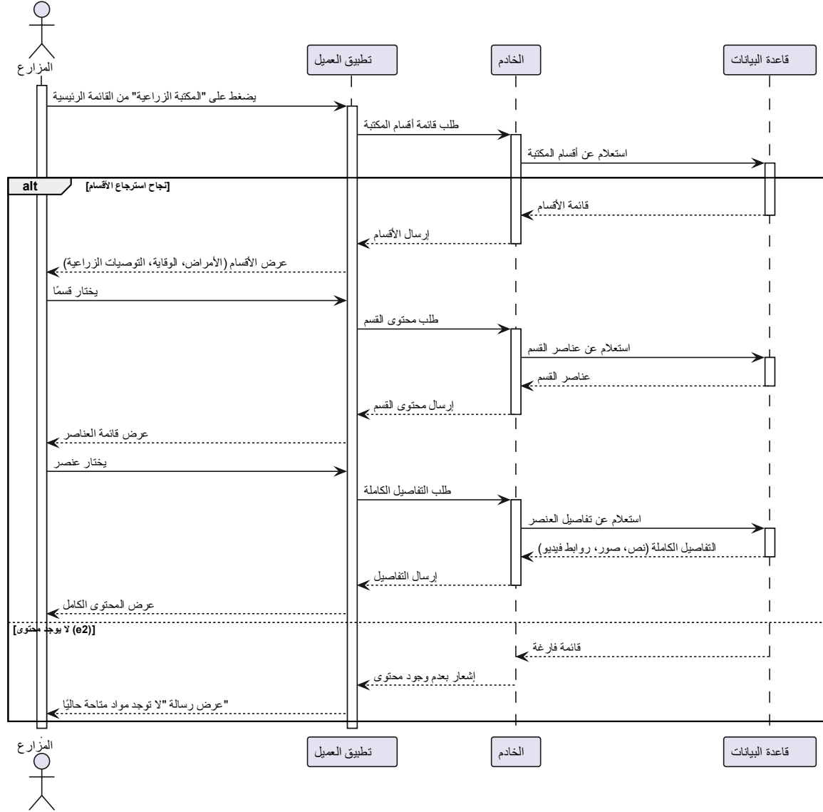
رسم توضيحي 1-13: مخطط تصفح المكتبة الزراعية
