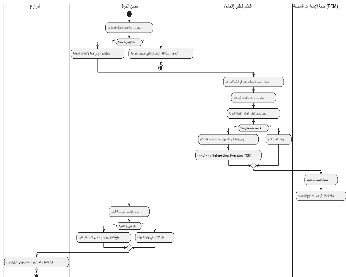
رسم توضيحي 8-1: مخطط النشاط ادارة الإشعارات وتنبيهات العلاج
