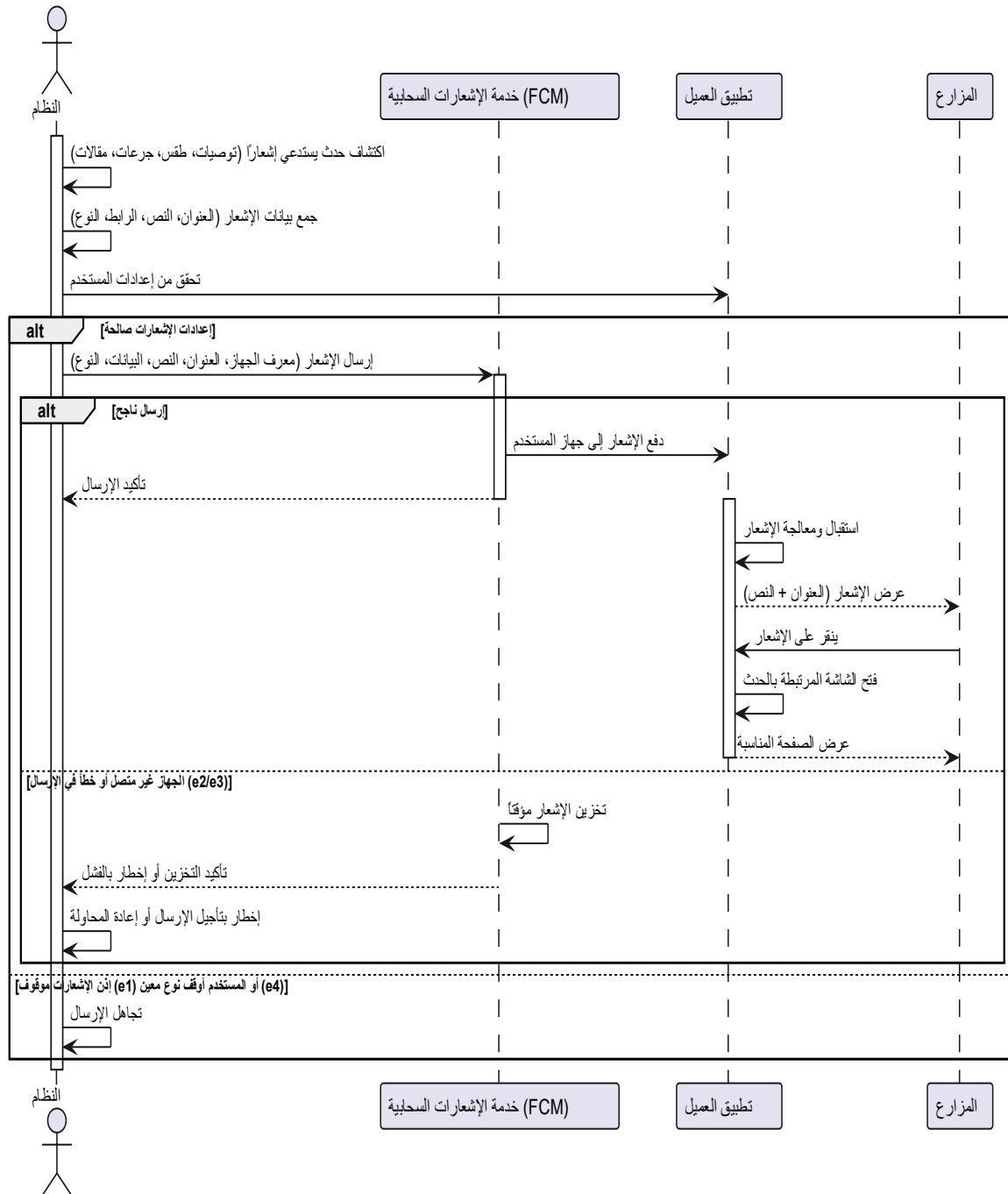
رسم توضيحي 1-14: مخطط إدارة الإشعارات وتنبيهات العلاج
